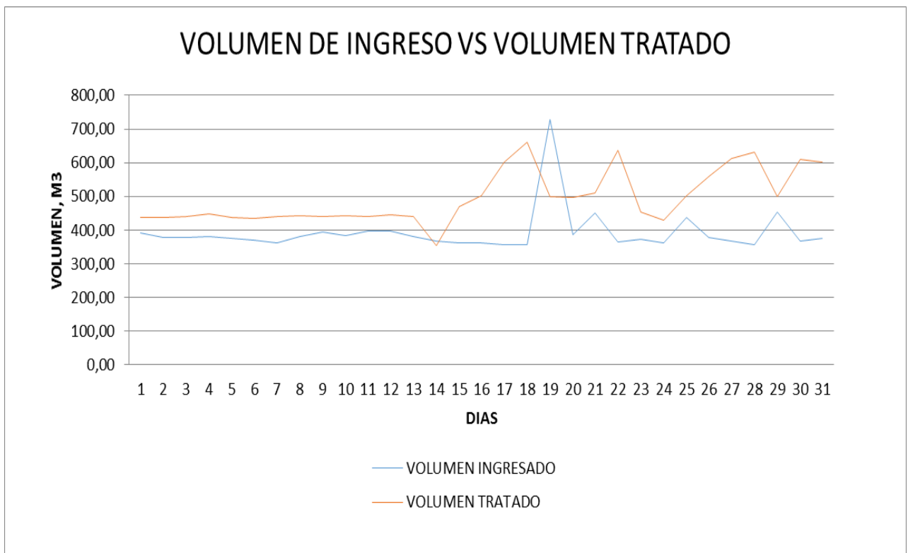
Diagrama 2: Volumen de ingreso vs volumen tratado
